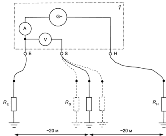
а) Линейное расположение электродов
