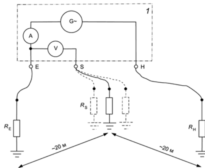
б) Расположение электродов треугольником
